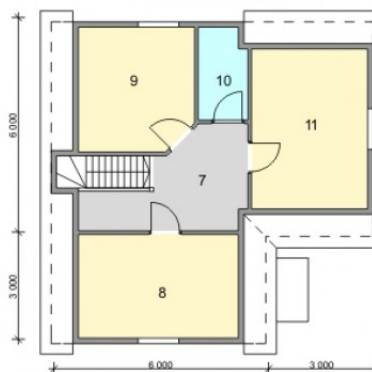
План мансарды
